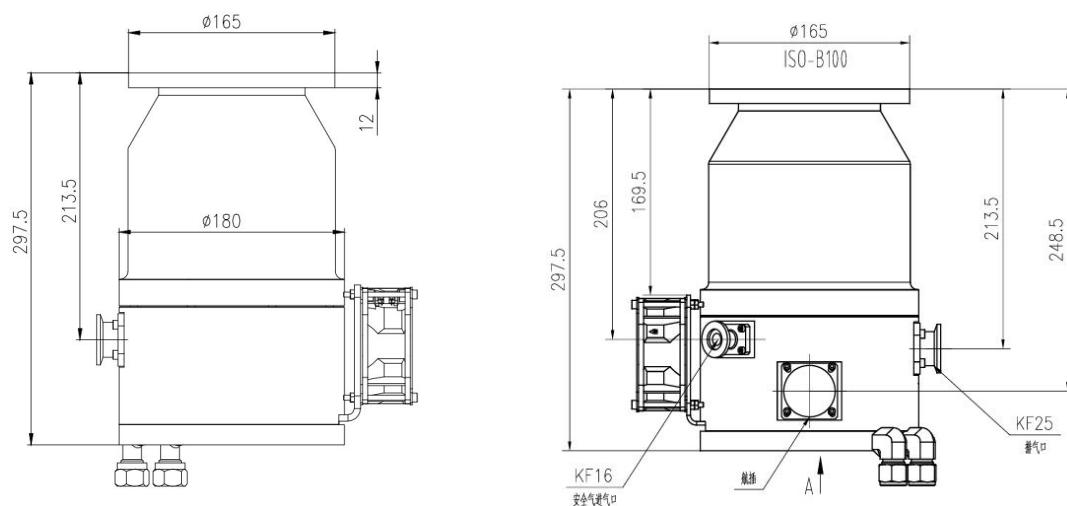
图 1.3 KTP-0304FC 风冷型磁悬浮分子泵侧视图
