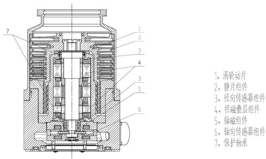
图 1.1 KTP-0304FC 型磁悬浮分子泵整机剖面图
