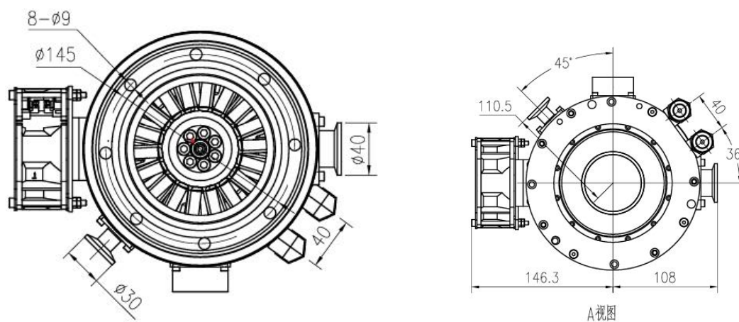
图 1.4 KTP-0304FC 风冷型磁悬浮分子泵俯视图与底视图
