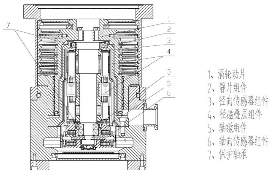
图 1.1 KTP-0304FC 型磁悬浮分子泵整机剖面图
