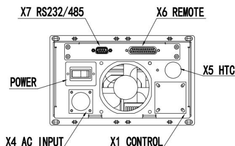
图 1.8 接口面板示意图
