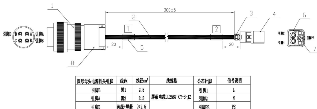
图 1.9 电源线缆及其连接说明
