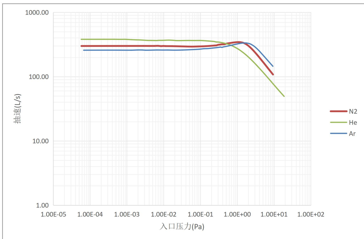
图 2.1 KTP-0304FC 抽速曲线
