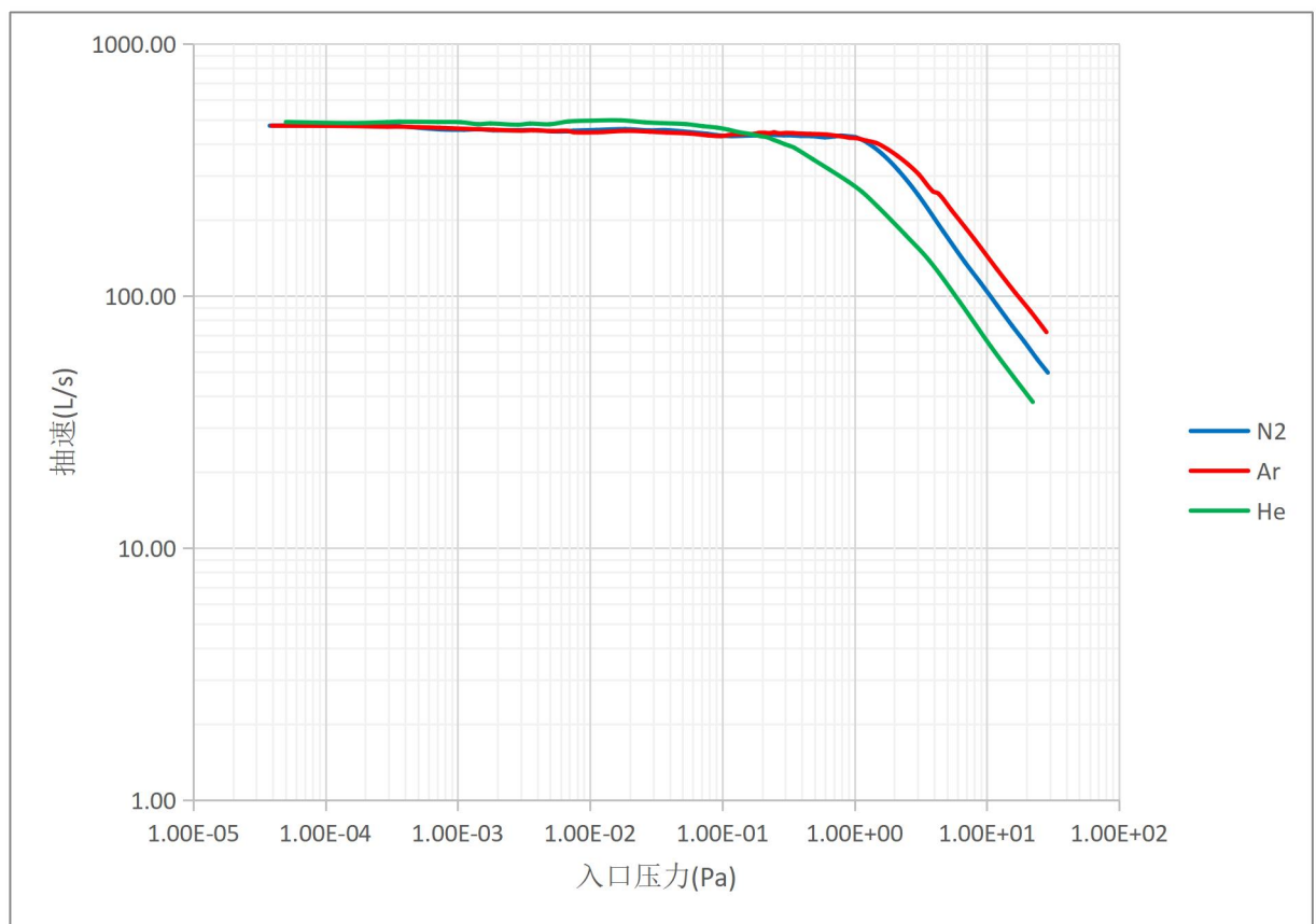
图 2.3 KTP-0454WC 抽速曲线
