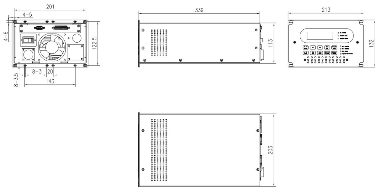
图 1.7 KTC-0106F 型磁悬浮分子泵控制器主要外形尺寸图
