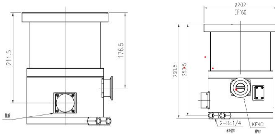
图 1.5 KTP-0454WC 水冷型磁悬浮分子泵侧视图
