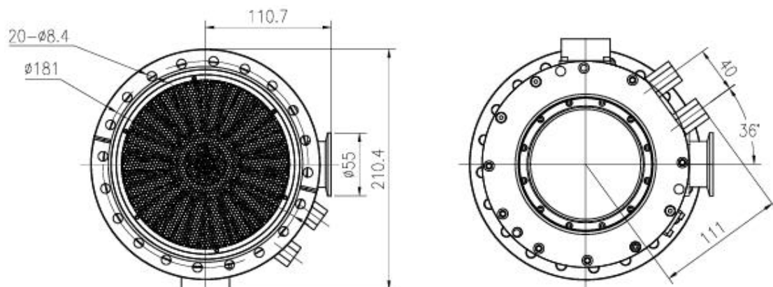
图 1.6 KTP-0454WC 水冷型磁悬浮分子泵俯视图与底视图
